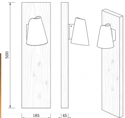
POST: 500mm (H) x 185mm (W) x 45mm (D) FITTING: 177mm (H) x 125mm (W) x 130mm (D)
